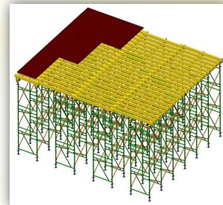
Стойка опорная телескопическая
