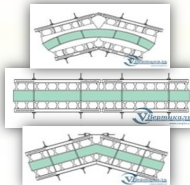
Балочно-ригельная опалубка
