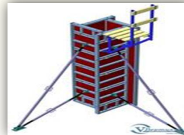
Опалубка колонн универсальная
