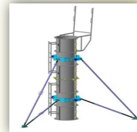
Колонна круглая
